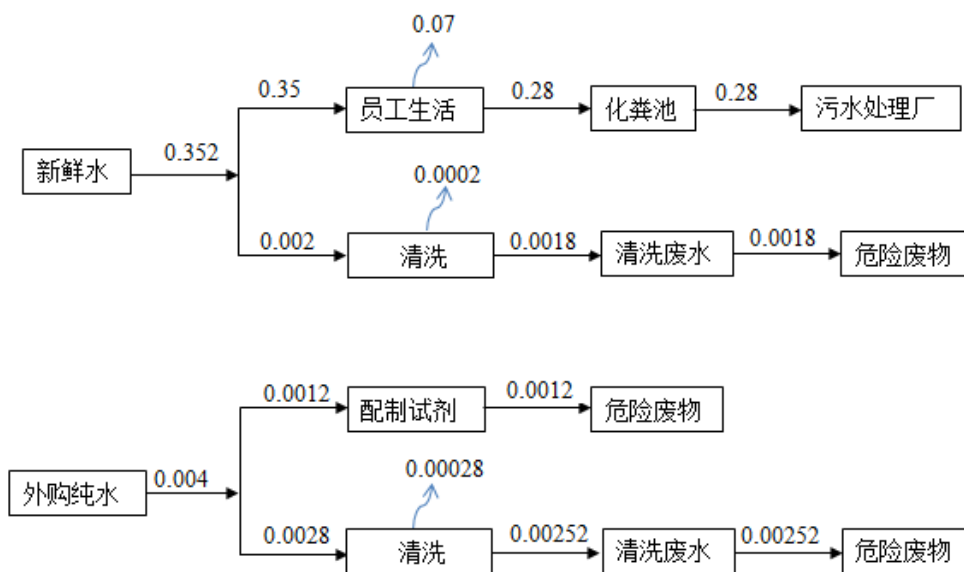
图1 项目水源平衡图 (单位: \text{m}^3/\text{d} )
